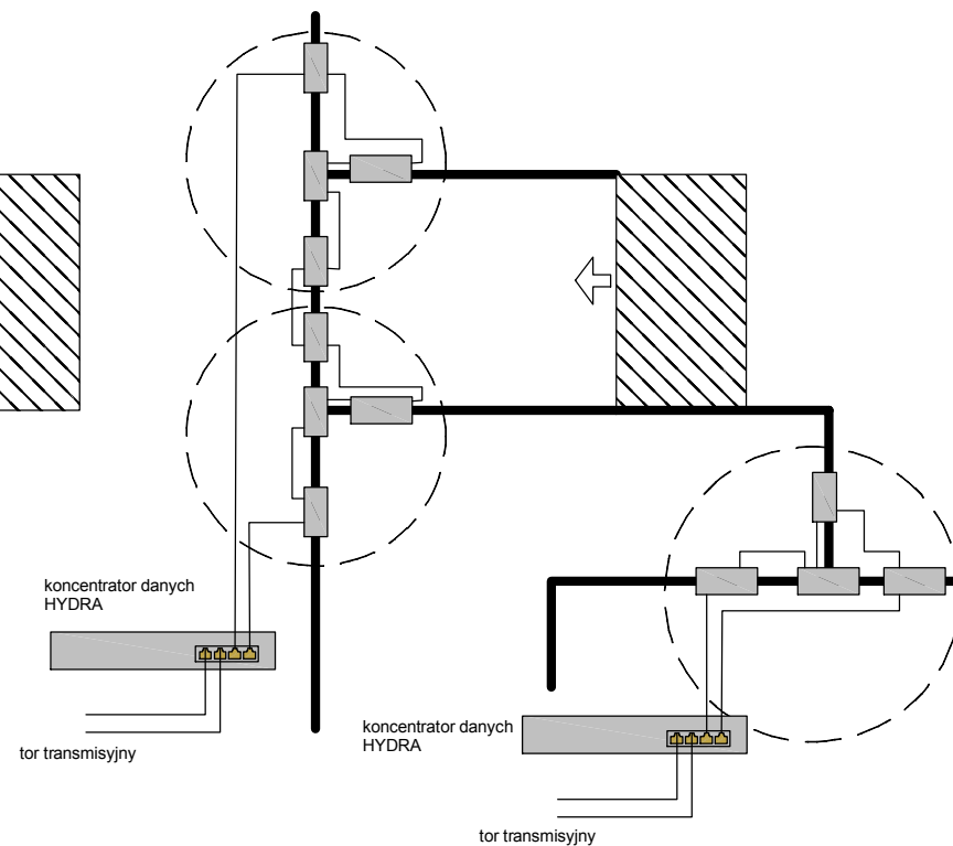
Przykładowa konfiguracja bramki rozmiszczenie czytników TGATE dla ścian przewietrzanych systemu na "Y"
