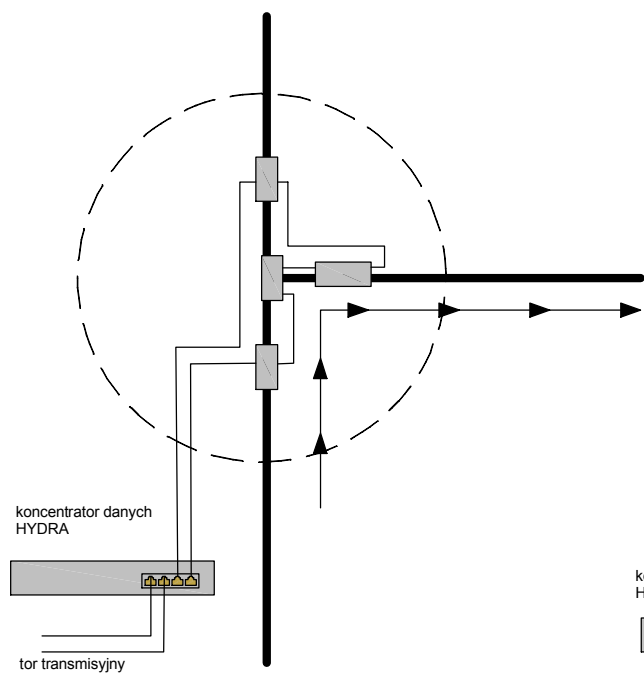
Przykładowa konfiguracja bramki typu T rozmiszczenie czytników TGATE dla drążonego wyrobiska
